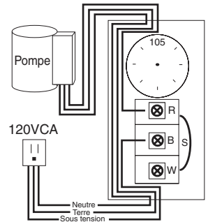
Câblage de l'aquistat Utilisez l'Aquistat Honeywell (Modèle L6006A ou L6006C)
